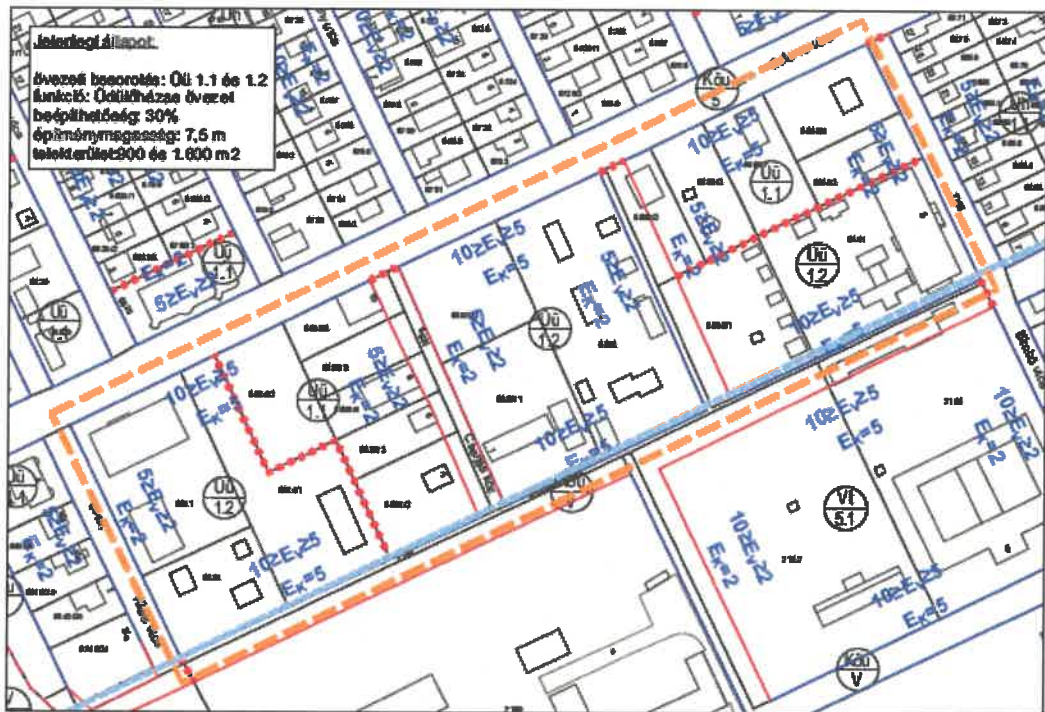
JELENLÉGI ÁLLAPOT
