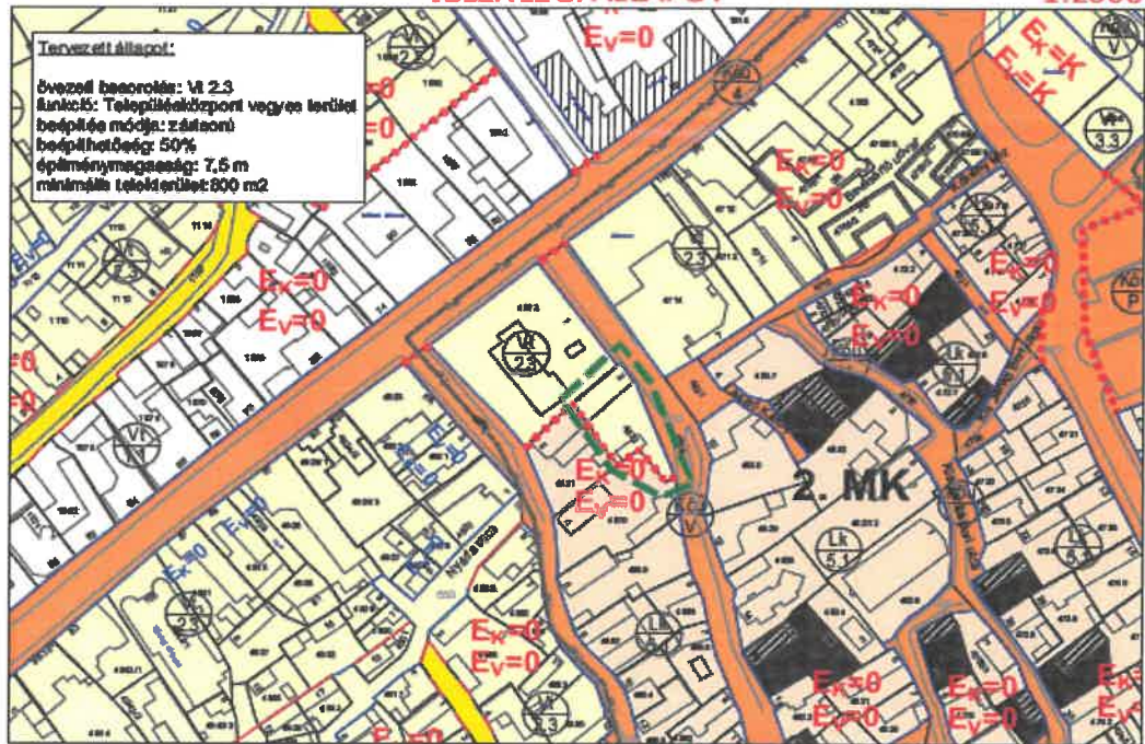
TERVEZETT MÓDOSÍTÁS
