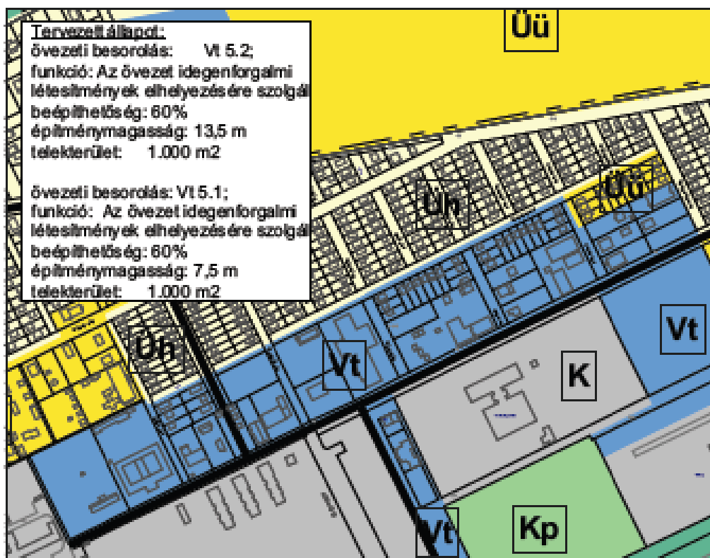
TERVEZETT ÁLLAPOT
